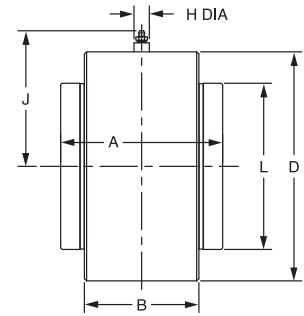
B-1 UNIT
