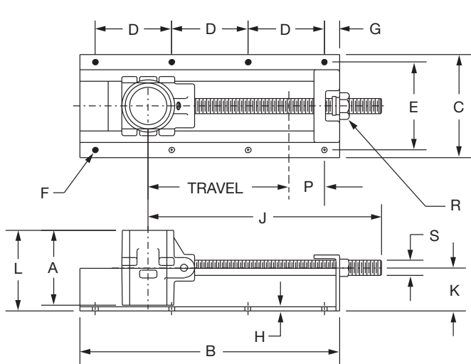
TYPE TUA
